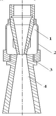
Şəkil1. İnjektor: 1- diffuzor; 2- injektor; 3- yarıqlar; 4- saplo.
