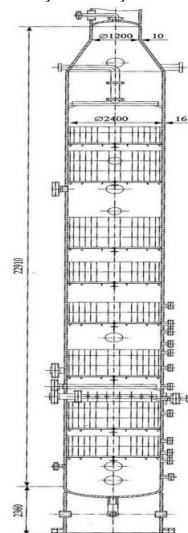
Şəkil 3. Müasirləşdirilmiş ekstraksiya kalonu.
