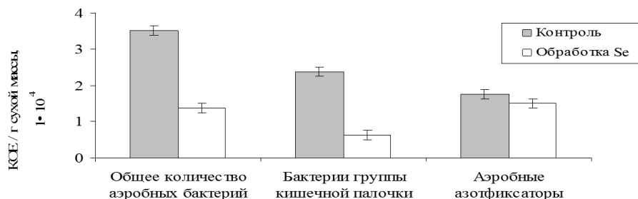
Рисунок 1 - Соотношение бактерий группы кишечной палочки, аэробных бактерий, усваивающих органический азот, и аэробных азотфиксаторов на контрольных и обработанных селеном семенах фасоли сорта «Сакса без волокна 615».
