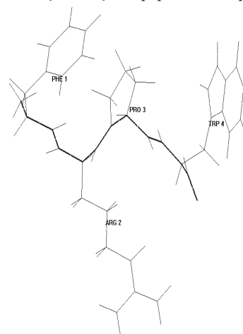
Şəkil 1. a) Phe-Arg-Pro-Trp tetrapeptidinin ən aşağı enerjili konformasiyaların ikiüzlü bucaqlarının və nisbi enerjilərinin qiymətləri cədvəldə göstərilmişdir; b) B_1B_{22}RB_1 konformasiyasının bucaqları əsasında modelləşdirilmiş tetrapeptidin fəza quruluşu
