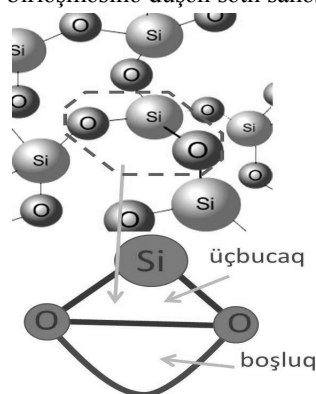
Şəkil 2. Bir \text{SiO}_2 birləşməsinə düşən səth sahəsinin hesablanması
