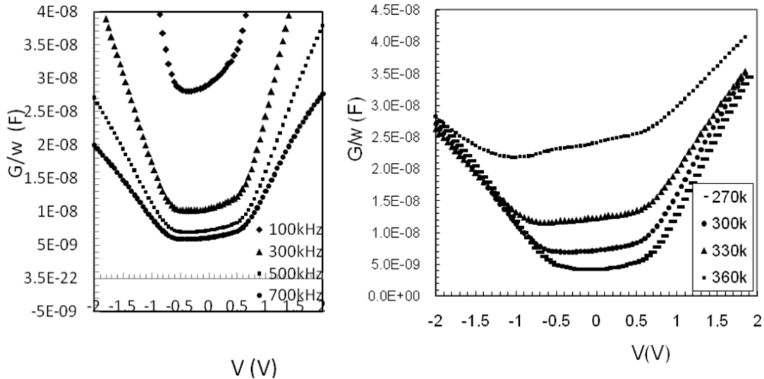
Şekil3. Kondüktans-Gerilim G/w -V ölçümleri oda sıcaklığında farklı frekanslarda (100 kHz-700 kHz) ve farklı sıcaklıklardaki (500 kHz frekansda) grafikleri.
