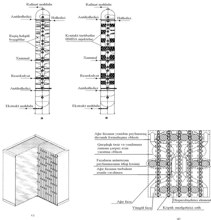
Şəkil 2. Ekstraksiya kalonları və onların daxili görüntüləri: a) əvvəlki ekstraksiya kolonu, b) yenilənmiş ekstraksiya kolonu, v) blokun ümumi görünüşü, q) blokun daxili görünüşü.
