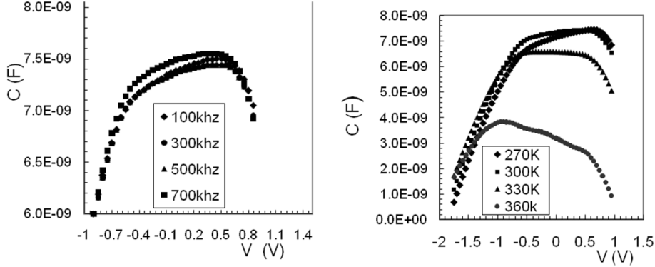
Şekil1. Diyodun farklı frekanslarda ve farklı sıcaklıklarda (500 kHz) kapasitans-gerilim (C-V) grafiki
