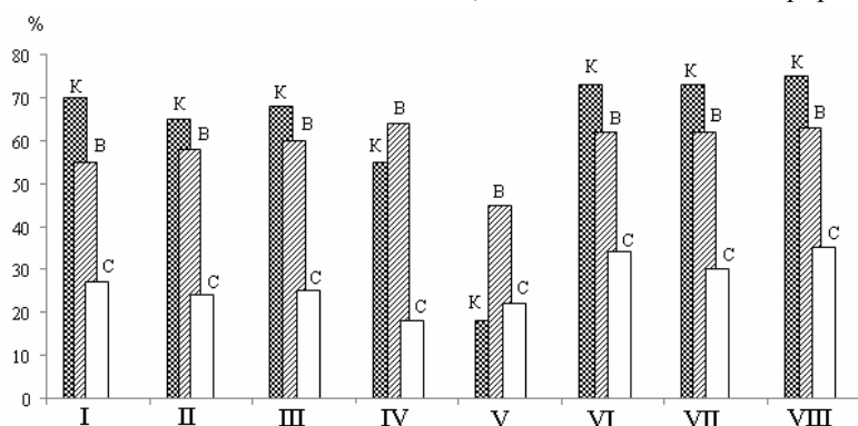
Рис. 1. Изменение активности Pt-Ga-M-O/HNa-ЦБМ в зависимости от природы оксидов РЗЭ.
