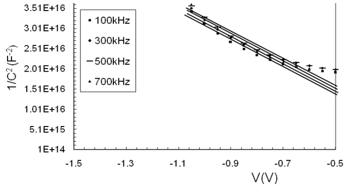
Şekil2. Diyodun oda sıcaklığında değişik frekanslardaki 1/C^2 -V değişim grafiki
