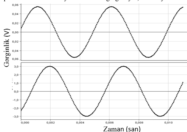
Şəkil 2. DataStudio proqramı vasitəsilə dövrəyə verilən tam gərginliyin, və cərəyanın zamandan asılılıq qrafikləri
