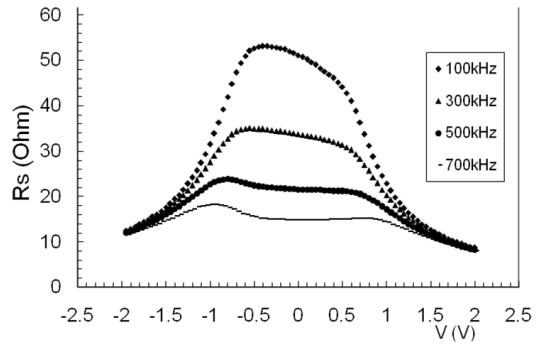
Şekil 4. Oda sıcaklığında farklı frekanslarda Au/p-GaAs Schottky diyodun
