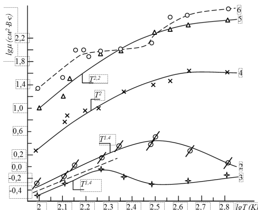
Şəkil. 1. Er_xSn_{1-x}Se bərk məhlullarında yükdaşıyıcıların yürüklüyünün temperatur asılılığı: 2- x=0,0010 , 3- x=0,0025 , 4- x=0,0050 , 5- x=0,0100 , 6- x=0,0250 .
