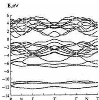
Şəkil. InGaTe_2 birləşməsinin zona quruluşu
