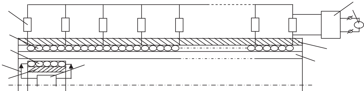
Şəkil 1. Paylanmış parametrlili böyük yerdəyişmələri ölçən qurğu
