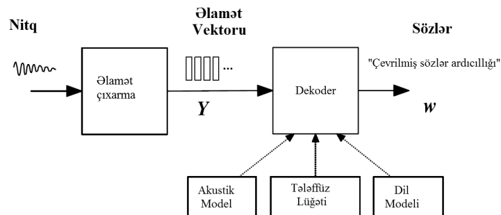
Şəkil 1. HMM əsaslı nitqi tanıma sisteminin işləmə prinsipi
