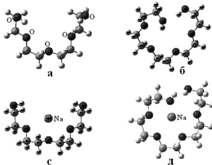
Рис. 1. Пространственные структуры моделей полиэтиленгликоля: (а) чистый PEG4, (б) чистый PEG5, (с) PEG4+Na, (д) PEG5+Na
