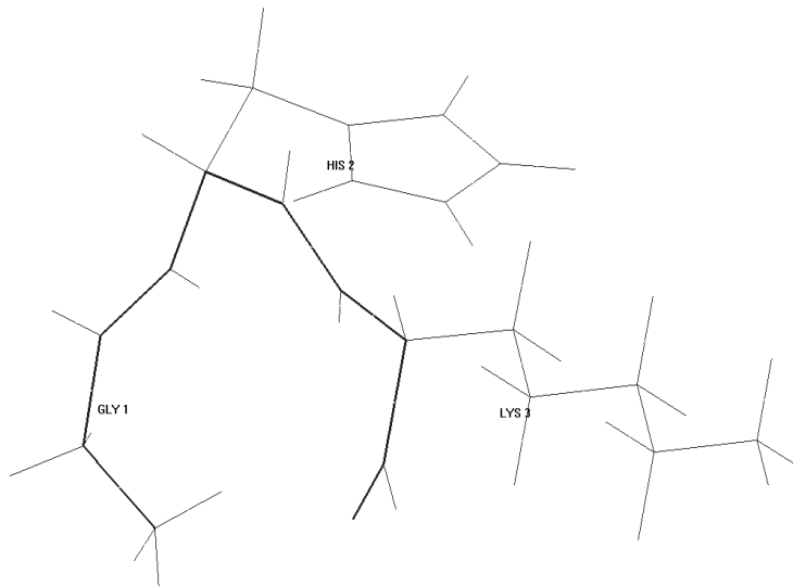
Şəkil 1. Gly-His-Lys tripeptid polyar mühiti üçün ən stabil konformasiyanın proyeksiyası.
