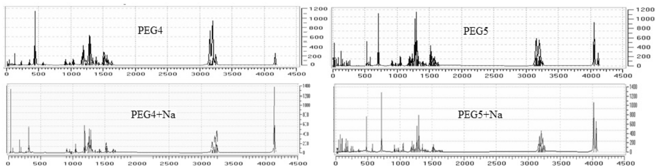
Рис.2. Теоретические спектры моделей исследуемых соединений
