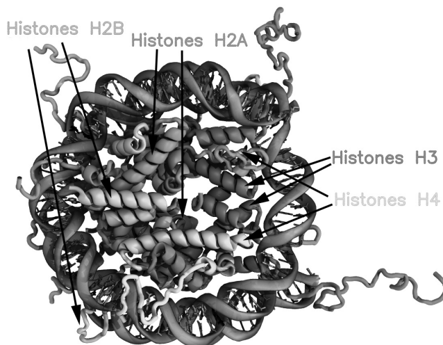
Рисунок 1. Молекулярная модель нуклеосомы: ДНК закручена вокруг 4 пар гистонов
