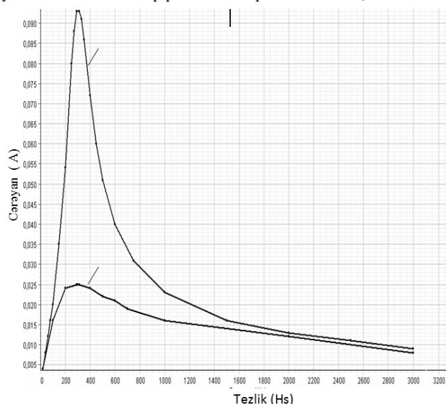
Şəkil 3. Cərəyanın tezlikdən asılılıq qrafiki 1- müqaviməti 10 Om, 2- 100 Om olan rezistorlar
