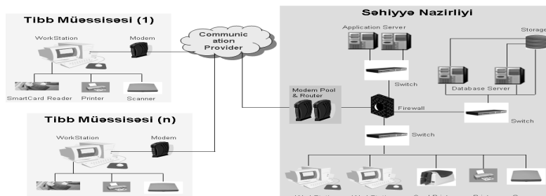
Şəbəkə Sxemi
