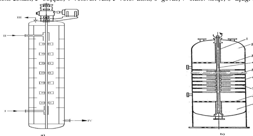
Şəkil 4. Rotorlu diskli kontaktör: a) I- xammal, , II- ekstragent, III- rafinat məhlulu, IV- ekstrakt məhlulunun axınları, b) 1-örtük val, 2- yuxarı çökmə zonası, 3- boşqab, 4- rotorun valı, 5- rotor diskli, 6- gövdə, 7- stator halqa, 8- aşağı çökmə zonası
