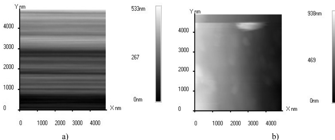
Şəkil 2. Monokristal səthinin həcmi AQM- təsviri: a) 3 həcm % TlInSe_2 ; b) 5 həcm % TlInSe_2
