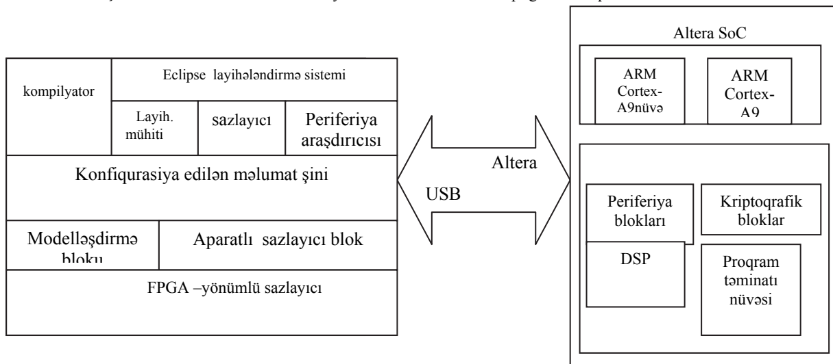
Şəkl.1. ARM DS-5™ sistemi ilə layihələndirilən SoC FPGA qurğunun əlaqələndirilməsi sxemi.
