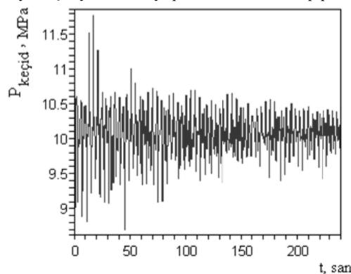
Şəkil 1. Mayenin konsentrik birləşdirilmiş boru kəmərlərində daxili borudan həlqəvi fəzaya keçid yerində təzyiqin zamandan asılılıq qrafiki
