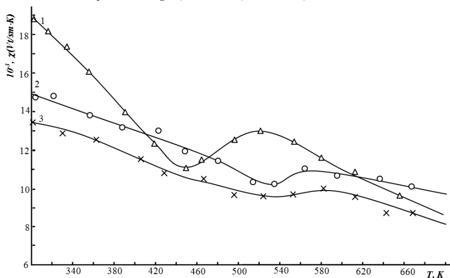
Şəkil 1. Pr_xSn_{1-x}Se sistem ərintilərinə istilikkeçiriciliyin temperatur asılılığı temperatur asılılığı. 1) x=0,000 ; 2) x=0,005 ; 3) x=0,010
