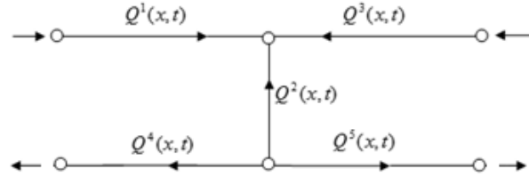
Рис.1. Схема нефтепровода с 5-тью участками
